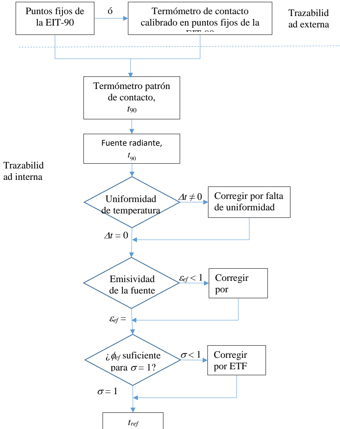
Fig. 3.1. Diagrama de flujo para obtener el valor de la temperatura de referencia cuando el termómetro patrón es uno de contacto y el que se calibra se encuentra ajustado a \varepsilon_{instr} = 1 .
