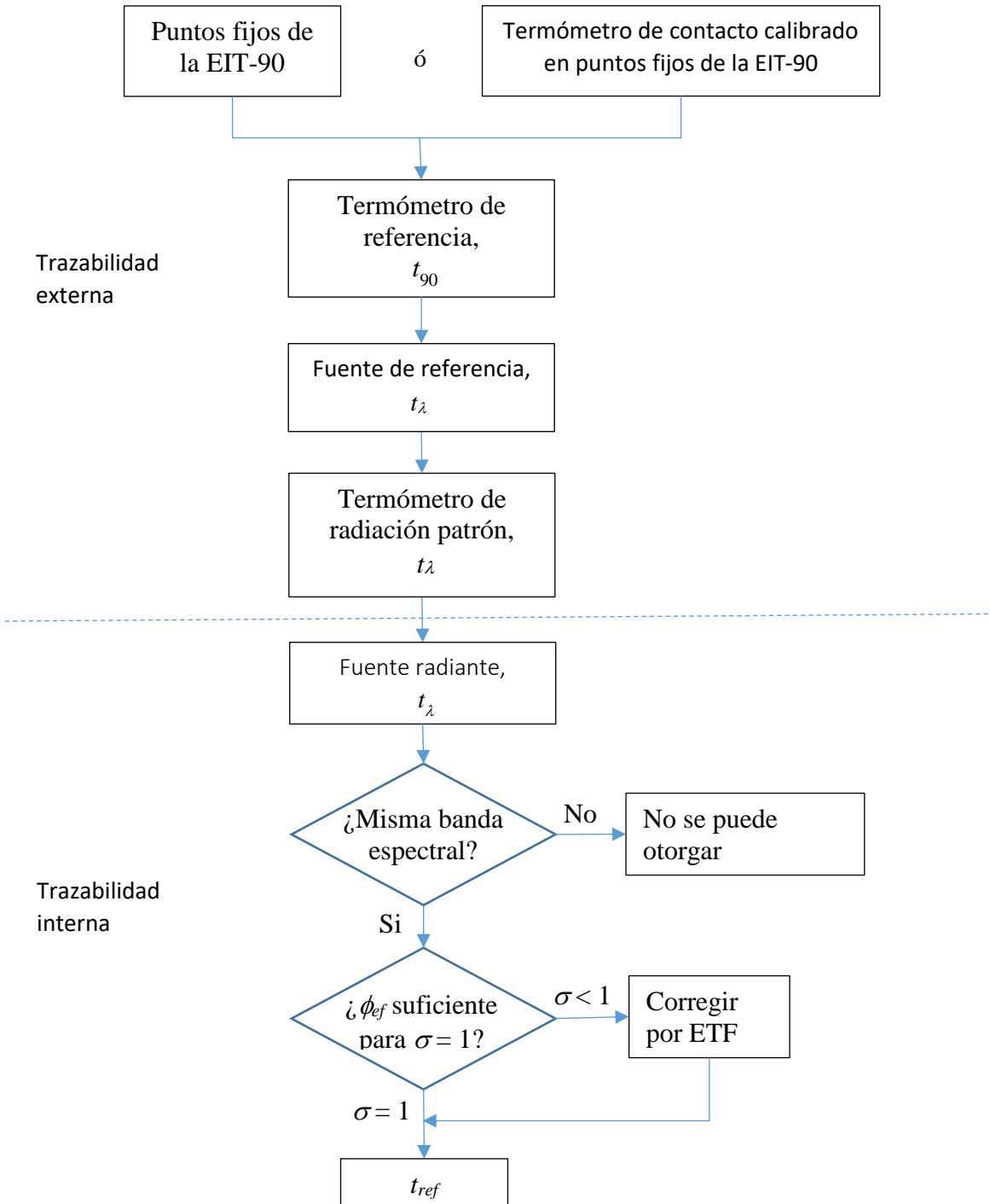
Fig. 3.3. Diagrama de flujo para obtener el valor de la temperatura de referencia cuando el patrón es una fuente calibrada con un termómetro de radiación.
